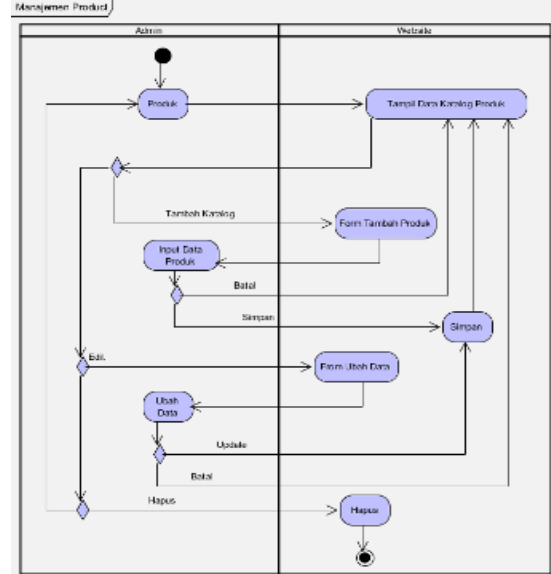
Gambar.8 Activity Diagram Manajemen Produk
