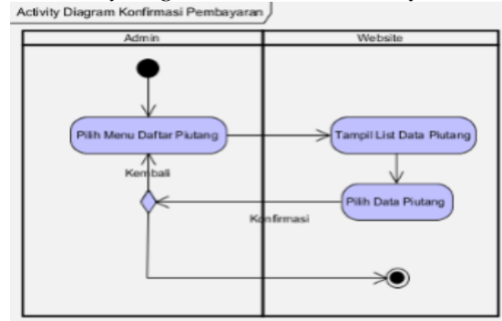
Gambar.9 Activity Diagram Input Pembayaran
