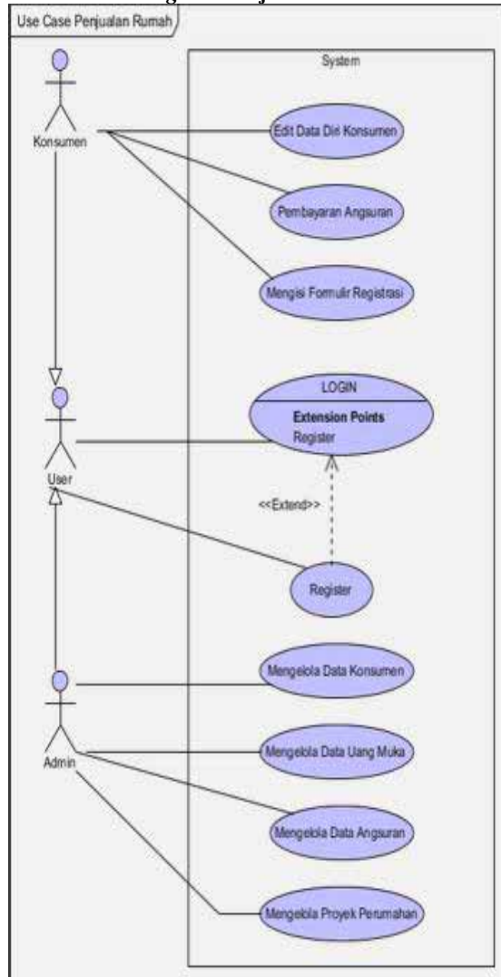
Gambar. 3 Use case Diagram Penjualan
