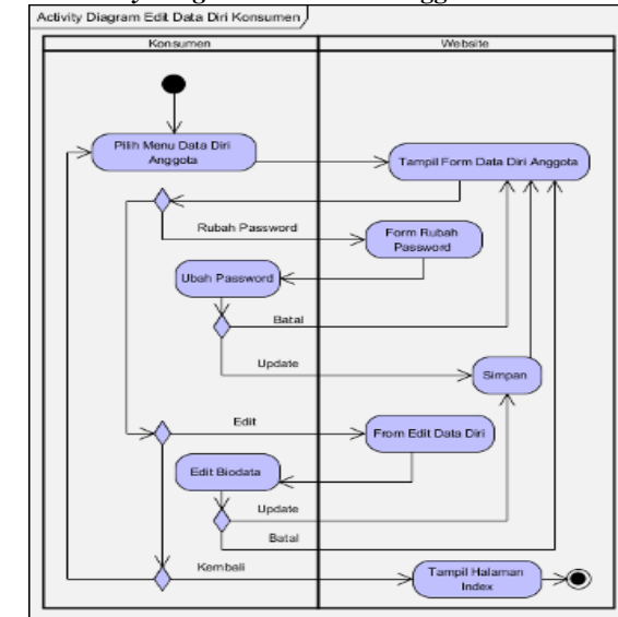
Gambar. 10 Activity Diagram Data Diri Anggota
