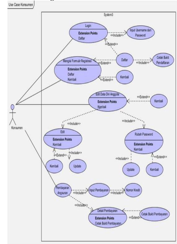
Gambar.5 Use case Diagram mengelola data akun konsumen
